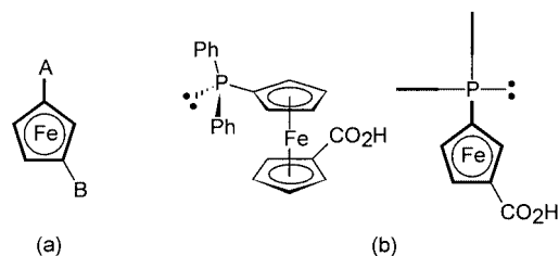
Scheme 20.
