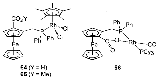
Scheme 19.
